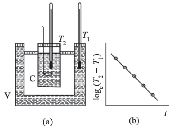
આકૃતિ 11.20 ન્યૂટનના શીતનના નિયમની ચકાસણી
