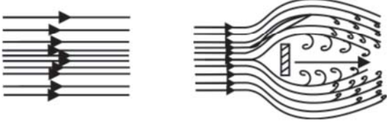
આકૃતિ 10.8 (a) તરલના વહન માટેની કેટલીક ધારારેખાઓ (b) જોશમાં નીકળતી હવા વહનને લંબરૂપે મૂકેલ સપાટ તકતીને અથડાય છે. આ પ્રક્ષુબ્ધ વહનનું ઉદાહરણ છે.
