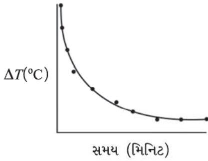
આકૃતિ 11.19 સમય સાથે ગરમ પાણીનું શીતન દર્શાવતો આલેખ
