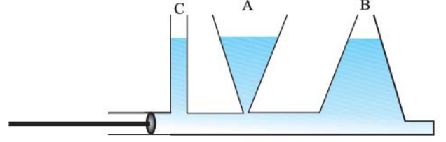
આકૃતિ 10.6(a) જ્યારે પાત્રમાંના તરલ પર કોઈ બાહ્ય દબાણ લગાડવામાં આવે ત્યારે તે બધી દિશામાં સમાન રીતે પ્રસરણ પામે છે.
