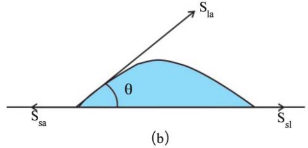
આકૃતિ 10.19 આંતરસપાટીઓમાંના તણાવ અને પાણીનાં બુંદ (ટીપાં)નાં જુદા જુદા આકારો (a) કમળની પાંખડી પર (b) સ્વચ્છ પ્લાસ્ટિક પ્લેટ પર
