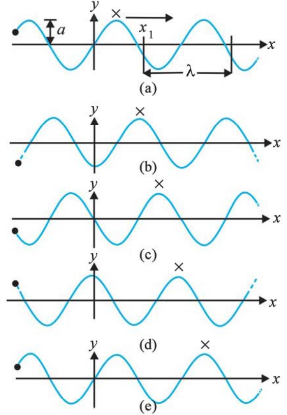
આકૃતિ 15.6 જુદા જુદા સમયે x -અક્ષની ધન દિશામાં ગતિ કરતું હાર્મોનિક તરંગ
