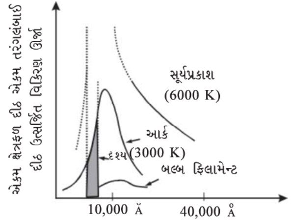
આકૃતિ 11.18: કાળા પદાર્થ માટે જુદાં જુદાં તાપમાને ઉત્સર્જિત ઊર્જા વિરુદ્ધ તરંગલંબાઈ
