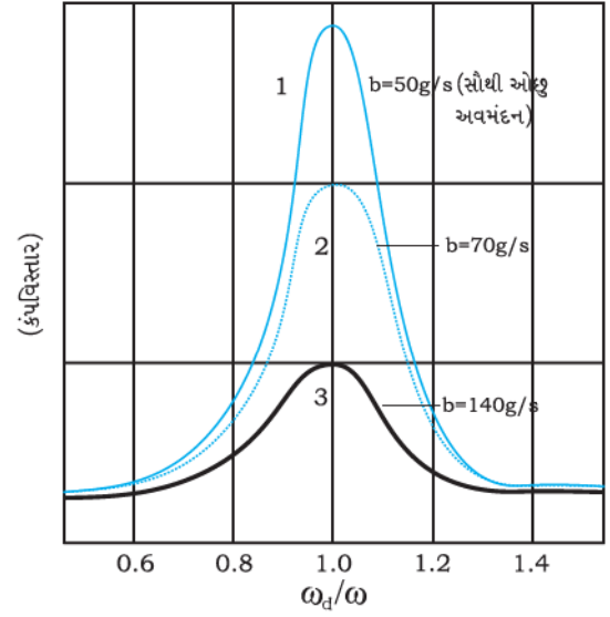
આકૃતિ 14.21 ચાલક બળની કોણીય આવૃત્તિના વિધેય તરીકે પ્રણોદિત દોલકનો સ્થાનાંતર કંપવિસ્તાર અનુનાદ શરત \omega_d / \omega = 1 આગળ કંપવિસ્તાર મહત્તમ છે. ત્રણ વક્રો તંત્રમાં પ્રવર્તતા જુદા જુદા અવમંદનને અનુરૂપ છે. વક્ર 1 અને 3 તંત્રમાં અનુક્રમે લઘુત્તમ અને મહત્તમ અવમંદનને અનુરૂપ છે.
