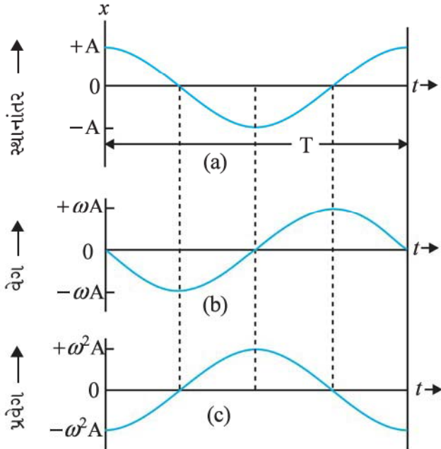
આકૃતિ 14.13 સરળ આવર્તગતિ કરતા કોઈ એક કણના સ્થાનાંતર વેગ અને પ્રવેગ સમાન આવર્તકાળનાં છે પણ કળામાં ભિન્ન છે.
