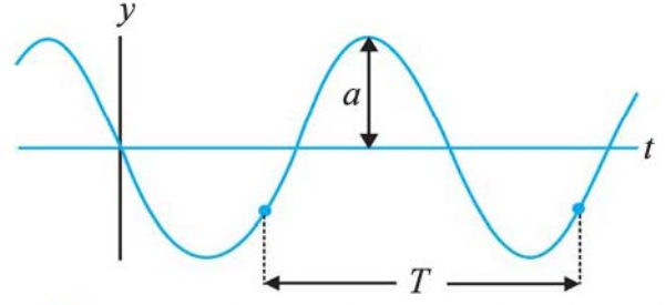
આકૃતિ 15.7 નિશ્ચિત સ્થાને રહેલ દોરીનો ખંડ જ્યારે તરંગ તેના પરથી પસાર થાય ત્યારે સમય સાથે કંપવિસ્તાર a અને આવર્તકાળ T સાથે દોલનો કરે છે.
